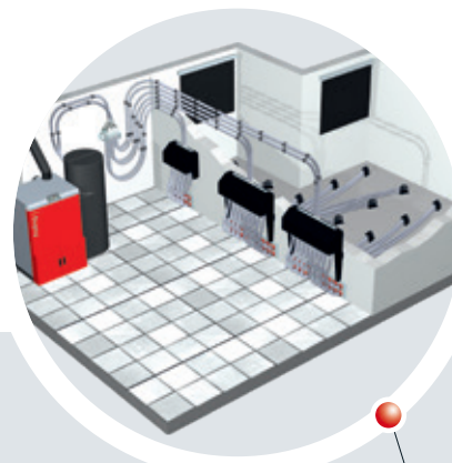
Système d'aspiration triple des granulés RS 4 / RS 8
