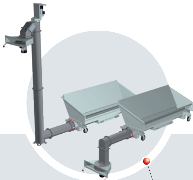
Systèmes de remplissage vertical et horizontal de silo
