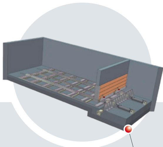
Extraction à bielles
