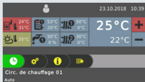
Vue d'ensemble du circuit de chauffage (écran d'accueil)
